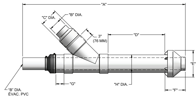
Figure 4-9 Dim. terminaison concentrique, modèles 400-500
