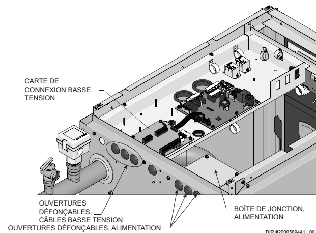
Figure 9-2 Câblage réalisé au chantier
