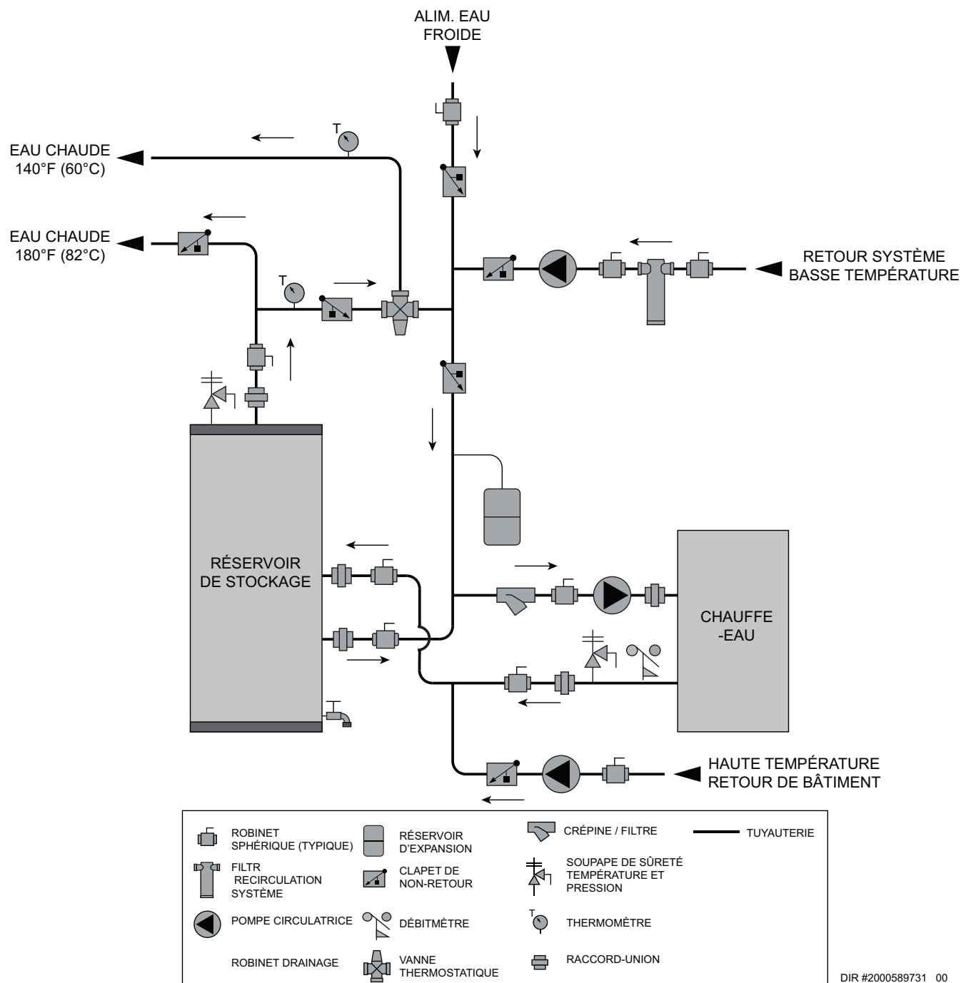
Figure 7-4 Un chauffe-eau, un réservoir (2 températures)
