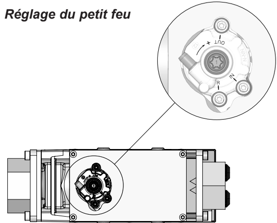
Figure 2-4 Réglage de la vanne du gaz: modèles 650 - 1000 Séries 110 - 111
